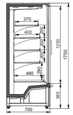
Hauteur 1700 mm Profondeur 700 mm ARC17XXXXX
