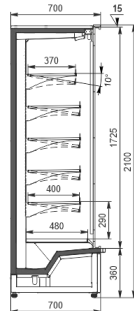
Hauteur 2100 mm Profondeur 700 mm ARC70XXXXX
