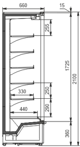
Hauteur 2100 mm Profondeur 660 mm ARC66XXXXX
