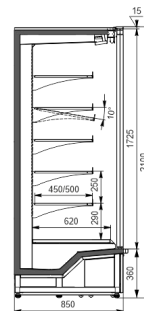
Hauteur 2100 mm Profondeur 850 mm ARC85XXXXX
